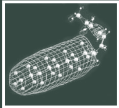
Modèle de la molécule RMNS entrant dans la composition d'ozane Hd.
